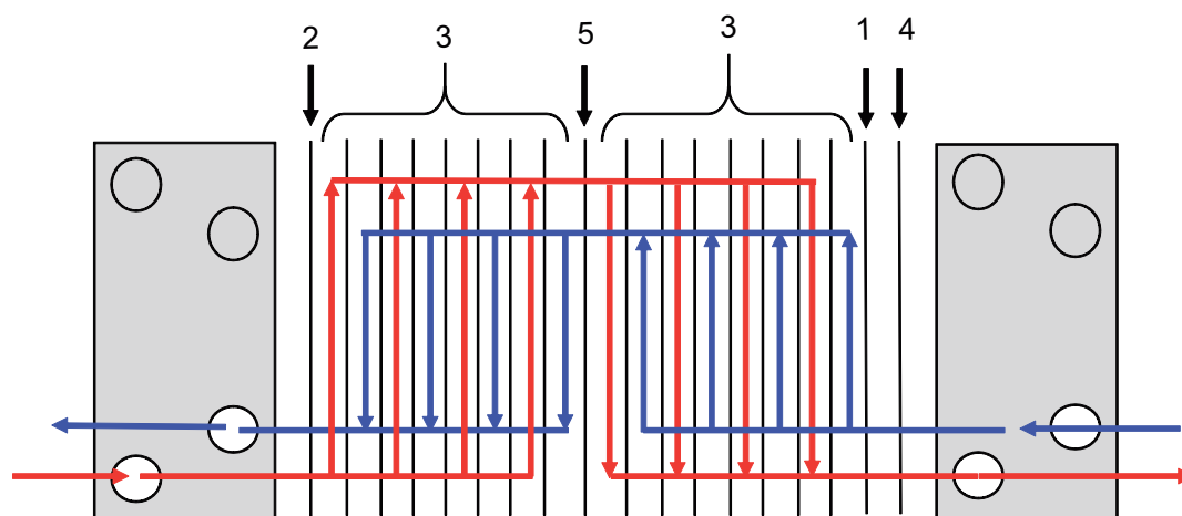
Obrázek 4: Příklad víceprůchodového nastavení.
