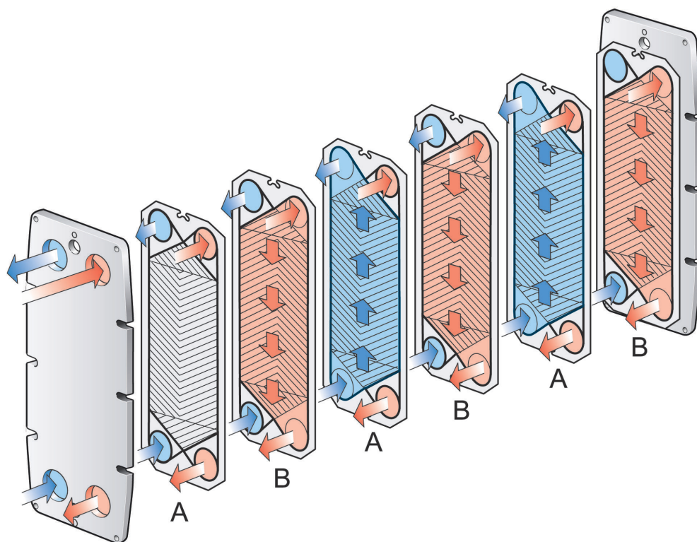
Obrázek 2: Princip souboru desek, uspořádání, těsnění ve styku se základní deskou.
