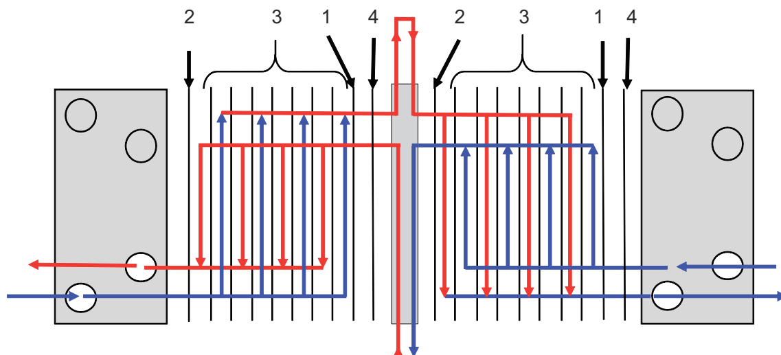
Figura 3: Ejemplo de una configuración de múltiples secciones.
