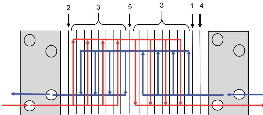
Figura 4: Ejemplo de una configuración de múltiples pasos.
