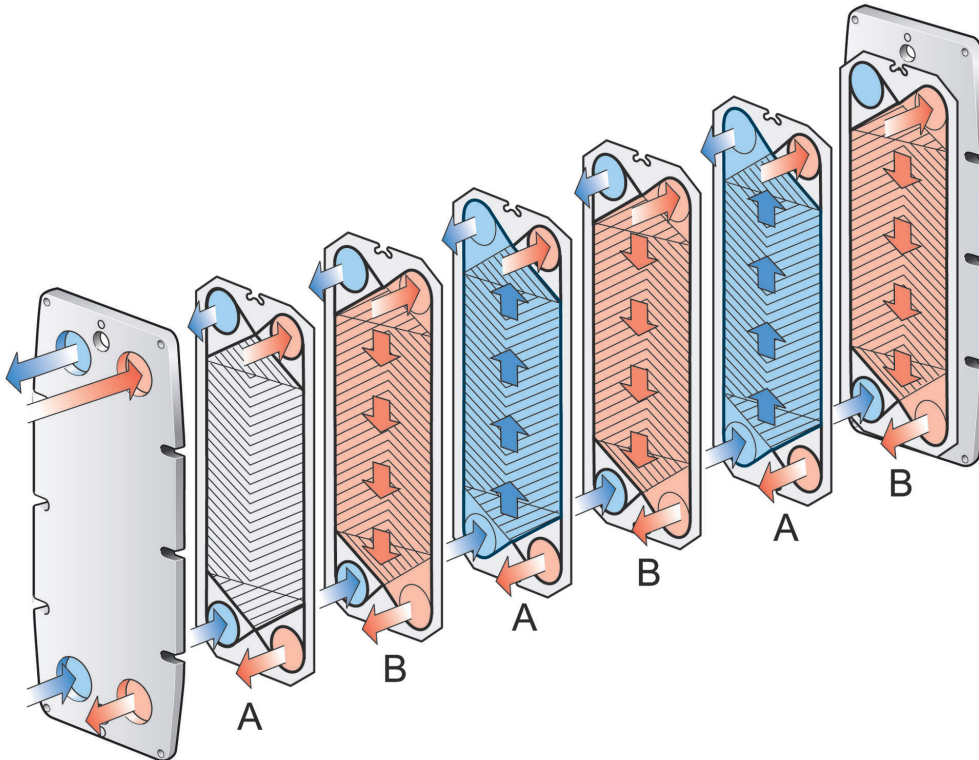
Figura 2: Principio de orden del conjunto de placas; juntas frente a la placa de bastidor.
