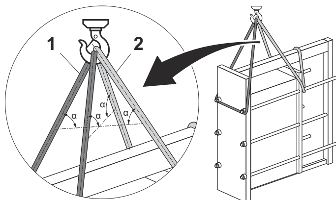
Figura 5: La ilustración muestra cómo colocar las eslingas de izar.
